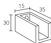
313011 Rosetta a muro Recess bracket Naissance murale
