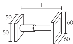
Raffhalter Alzapaño Przytrzymanie franki
