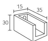
313012 Wandlager Soporte lateral Podkładka do muru
