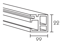
223100 Profilo Profile Profil Profil Perfil Profil
