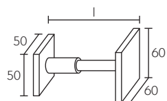
5130-- Fermatenda Holdback Porte-embrasse
