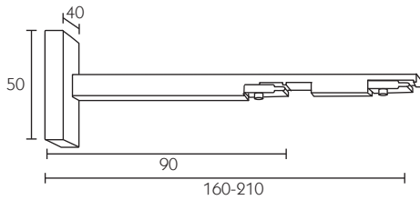
223317 Supporto doppio Double bracket Support double
