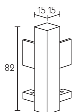
823312 Giunzione ad angolo Angle juncton Jonction à angle Ecke Verbinder Ângulo Łącznik kątowy
