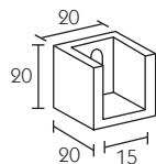
163001 Rosetta a muro Recess bracket Naissance murale Wandlager Soporte lateral Podkładka do muru
