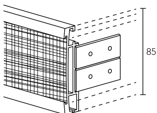
9231-- Angolare Angle Retour
