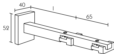
333517 Rita Supporto doppio
