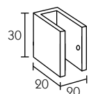
313003 Marcella Rosetta a muro
