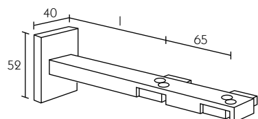
223437 Adele 353117 Clara Supporto doppio
