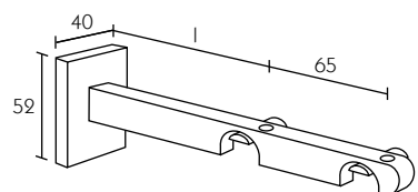
203345 Diva 20 Supporto doppio
